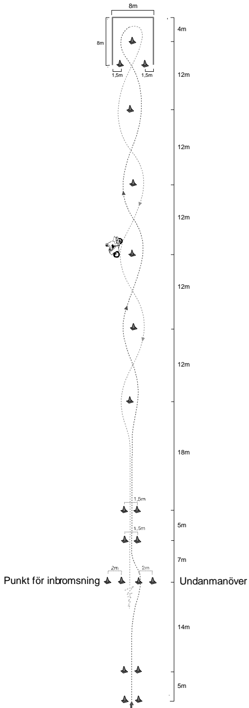
Figur 3. Manöverprovets högfartsdel
